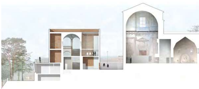
Sección transversal
