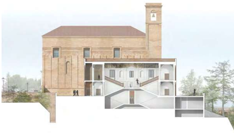
Sección longitudinal
